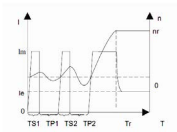
Рисунок 5-5 Пуск с поворотом
