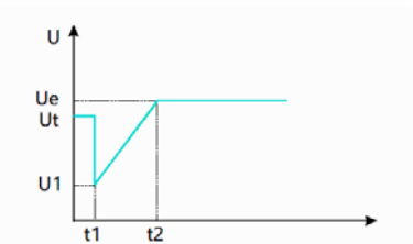
Рисунок 5- 4. Начало линейного изменения напряжения при скачке напряжения.
