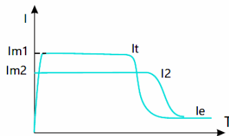
Рисунок 5-1 Пуск с ограничением тока
