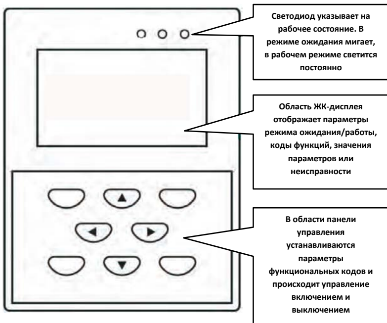
Рисунок 2-1 Панель управления
